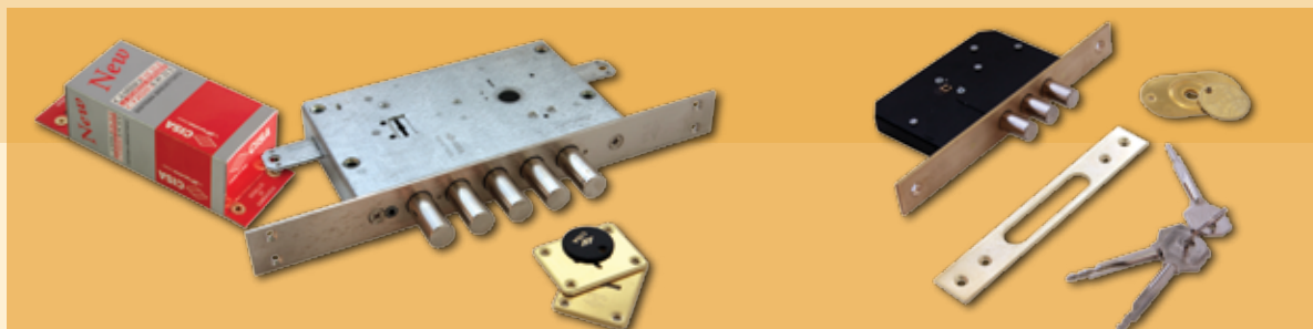
Yalla CISA 625 cheie tip seif, inchidere pe 3 laturi in 3 puncte, cu sistem de recodare, montaj cu cheie de service
