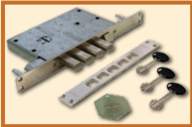
Broasca MOTTURA M 779 cheie tip seif, inchidere pe 3 laturi in 3 puncte
