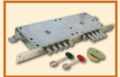
Broasca MOTTURA M 774 cheie tip seif, inchidere pe 3 laturi in 4 puncte+ sistem de autoblocare
