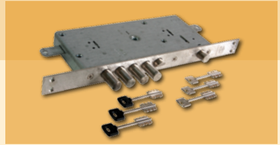
Broasca CISA 735 cheie tip seif, inchidere pe 3 laturi in 4 puncte + sistem de autoblocare
